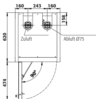
Draufsicht
