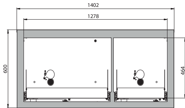
Frontalansicht
