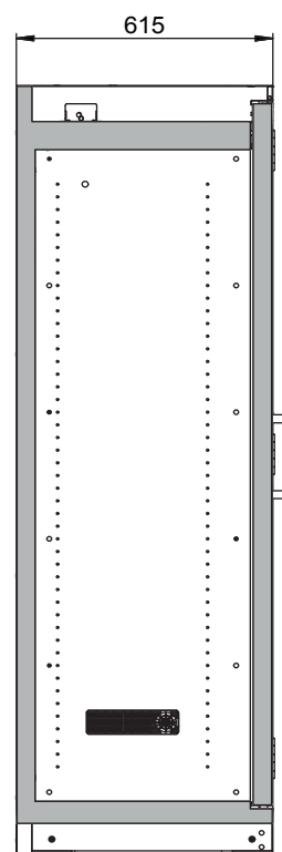
Vue latérale
