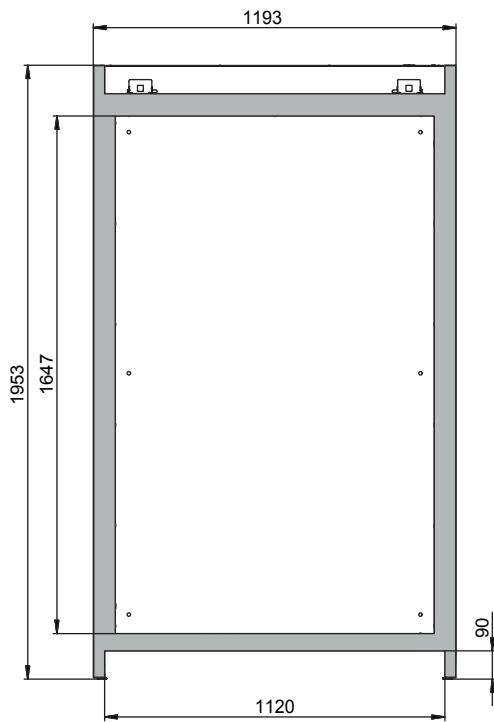
Frontalansicht
