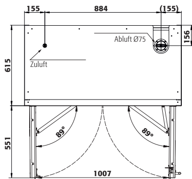
Draufsicht
