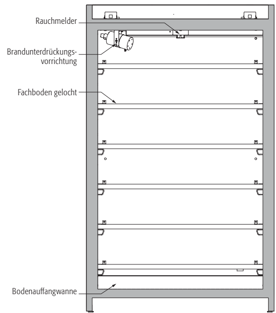
Schnittansicht
