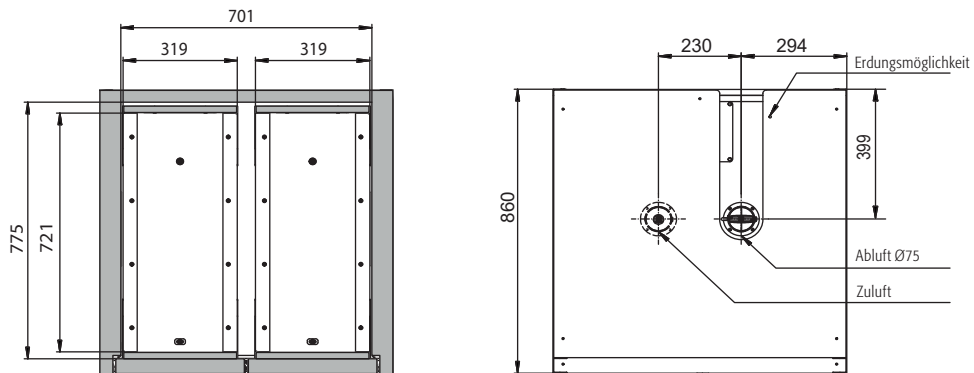
Draufsicht
